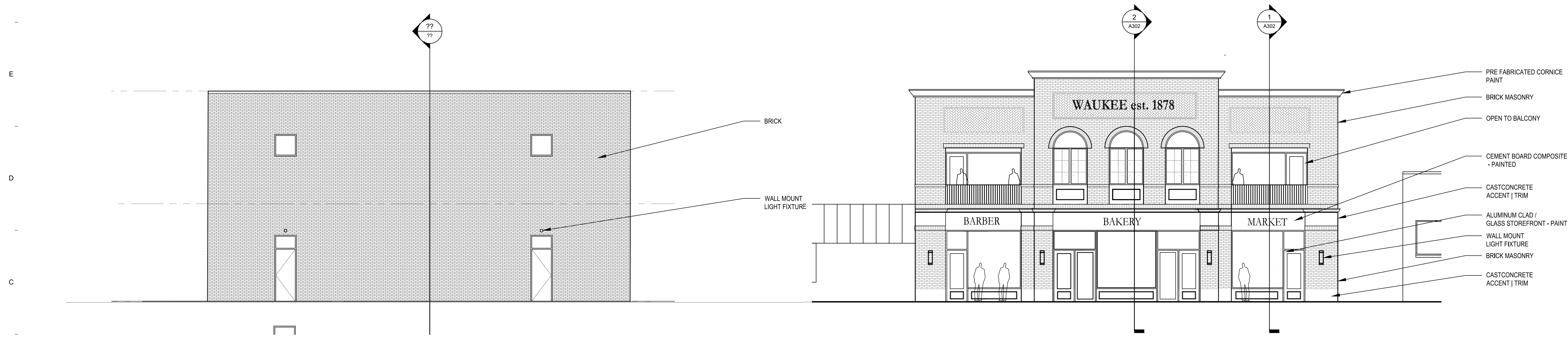
1 ELEVATION - WEST SCALE: 1/8" = 1'-0"
