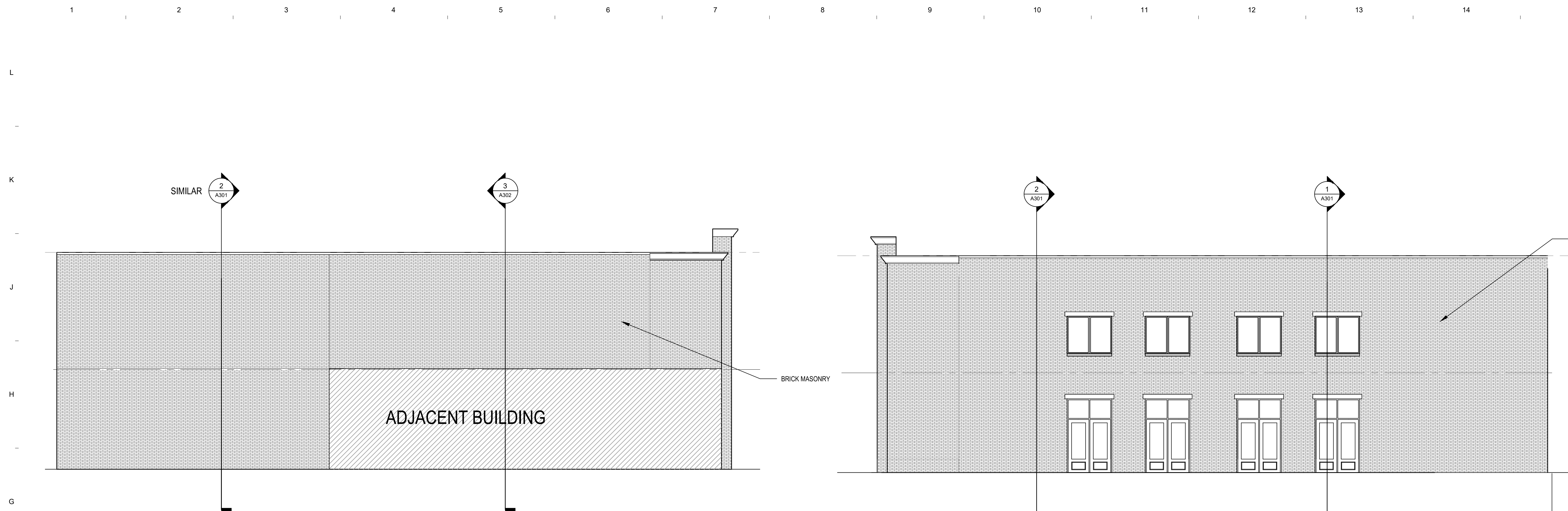
2 ELEVATION - SOUTH SCALE: 1/8" = 1'-0"
